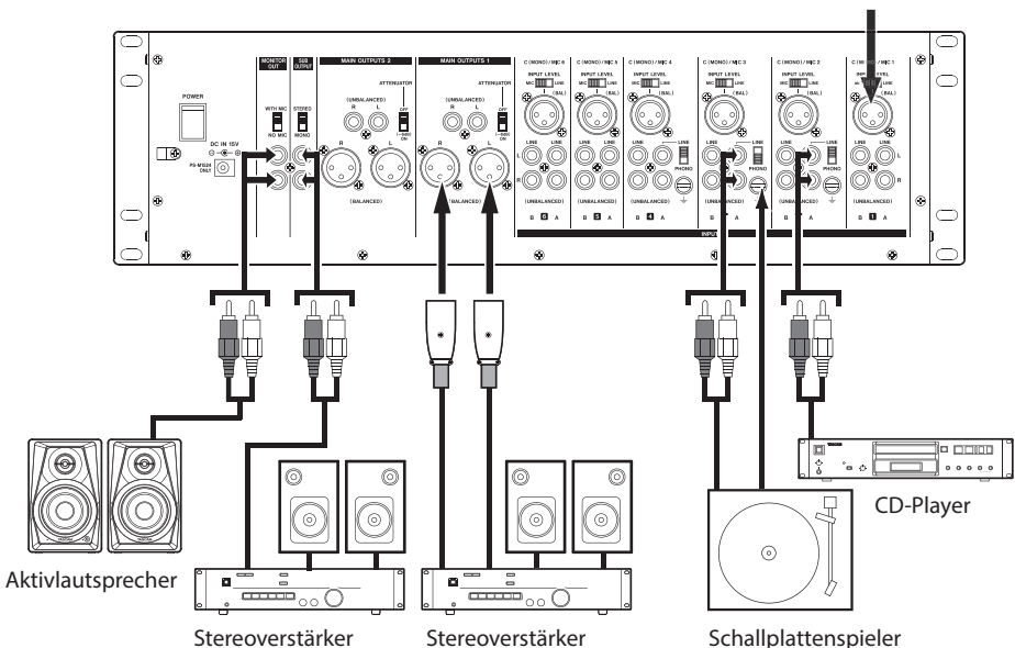
Anschlussbeispiel MZ-372
