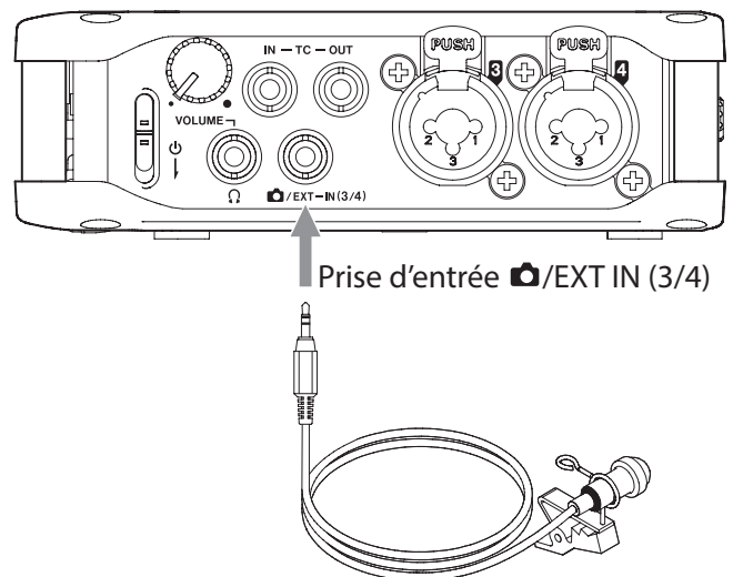
Micro nécessitant une alimentation par la prise (plug-in)
